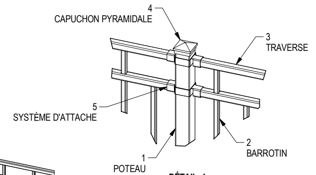
DÉTAIL 1 ÉCHELLE 1 : 10
