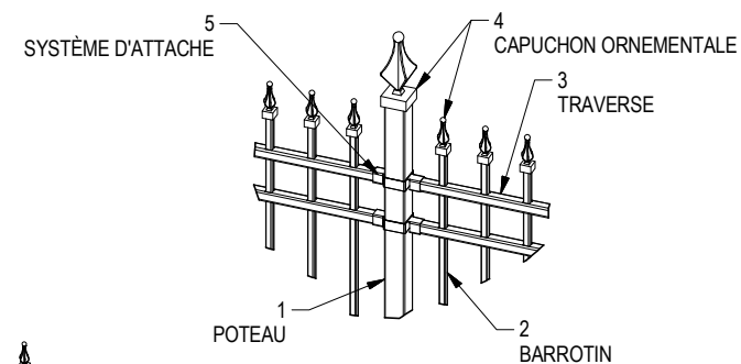
DÉTAIL 1 ÉCHELLE 1 : 16
